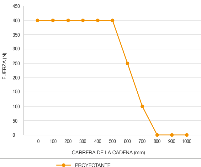
L40 Slim - 1000 - Capacidades de los actuadores para ventanas proyectantes
