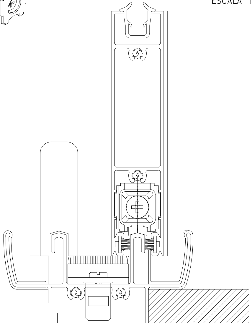
ESCALA 1:2
